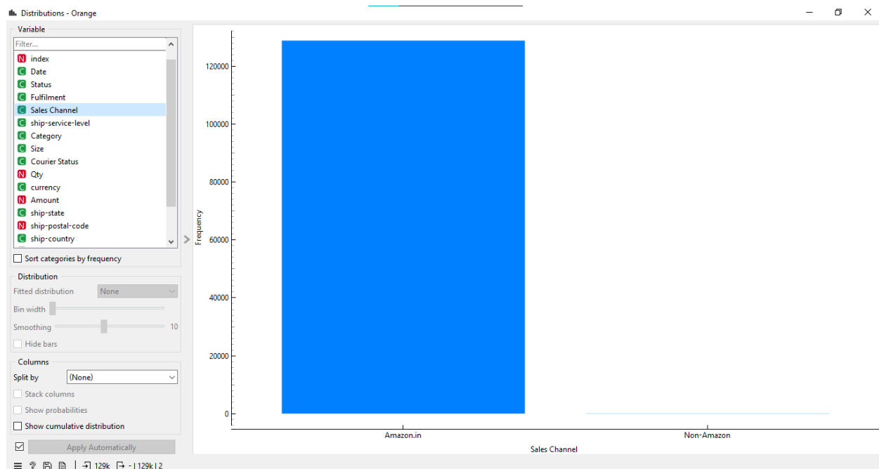
Рисунок 8 – Distributions
