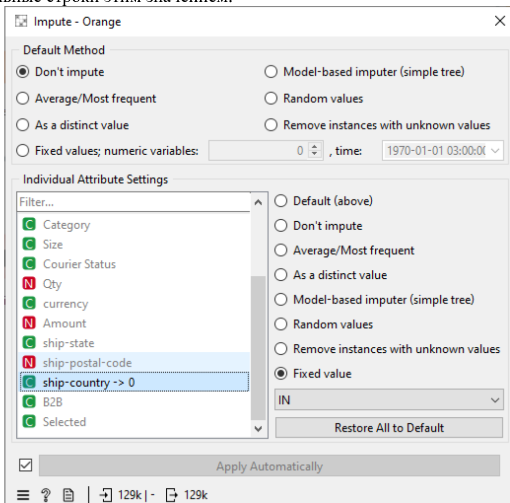
Рисунок 12 – Impute
